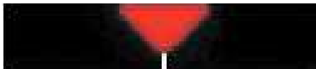
Незавершенный сварной шов, оставляющий зазор на вершине раздела кромок, который стимулирует появление коррозии
